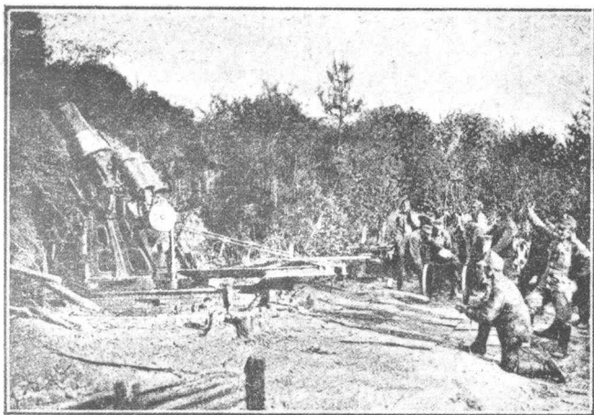
Найбільша австрійська важка гармата, 30,5 цм. »Мерзер« готовий до стрілу.
